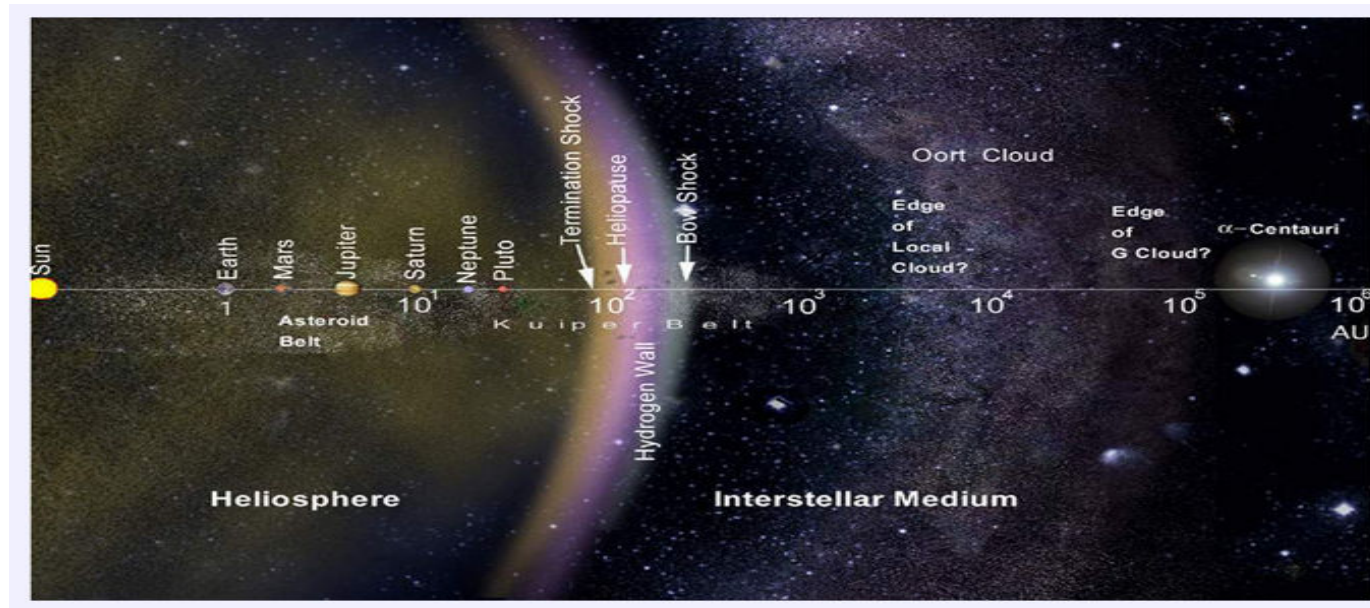
Ceinture de Kuiper Nuage de Oort
