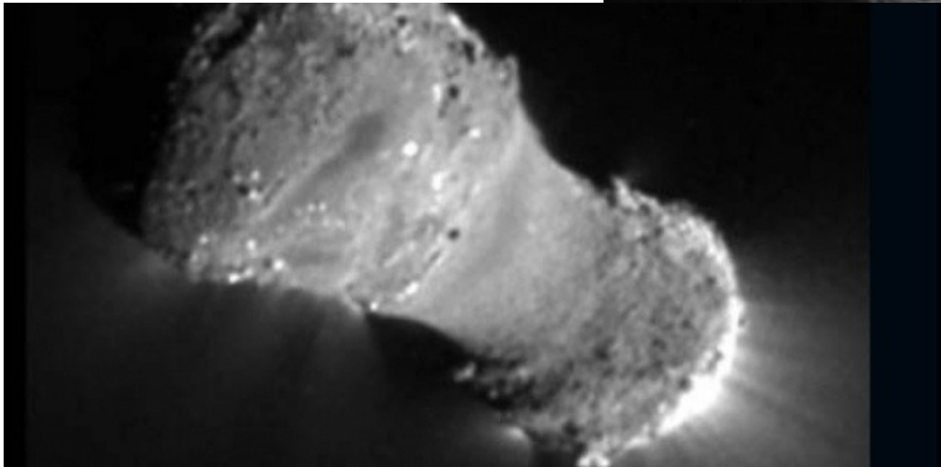
P/Hartley 2
